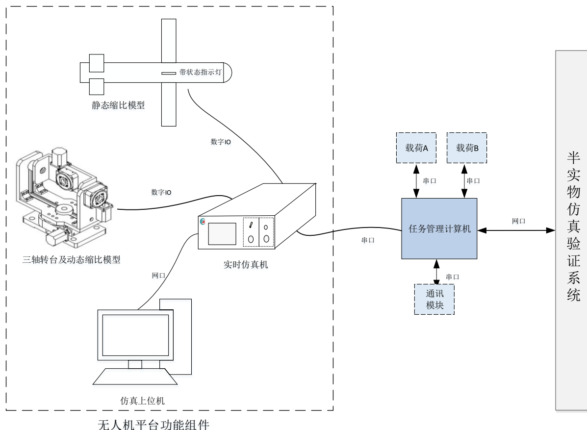
图 1 系统总体构成框图
